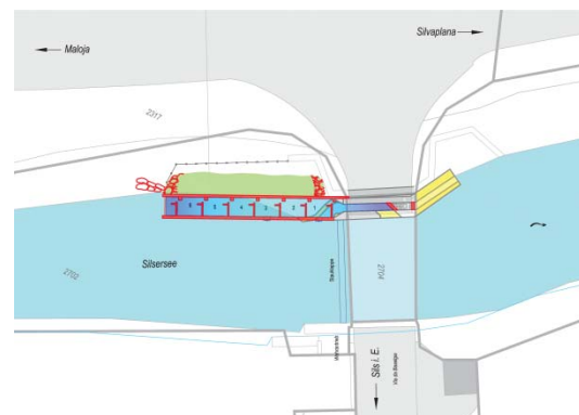
Projektskizze Fischschleuse
